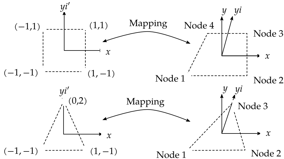
Figure 4-1. Isoparametric mapping if GLOBAL = 1
